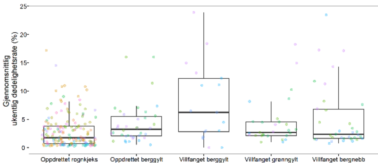
Figur 3: Gjennomsnittlig ukentlig dødelighetsrate på merdnivå. Datapunktene er farget etter lokalitet, og boksploTTene viser fordelingen av dødelighetsraten til hver av artene (se Figur 2 for fargekoden til lokalitetene).
