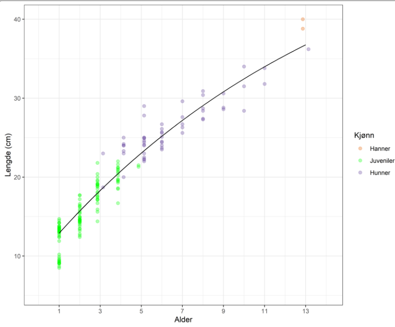
Figur 3: Berggylt alder versus lengde. Data fra bestandsundersøkelser Havforskningsinstituttet.
